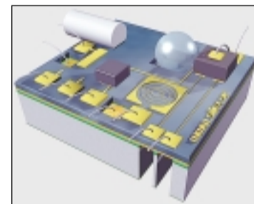
En mikrooptisk hybridbank för telekomindustrin. Banken är ett pre-fabricerat kiselsubstrat som fungerar som bärare för optiska komponenter som lasrar, detektorer, fibrer och linser samtidigt som diskreta komponenter integreras på chipet. Chipet är en standardprodukt som tagits fram av Silex Microsystems AB.
